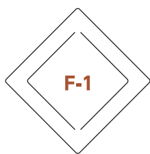
W20×H20mm 0.5R (内刃14mm×14mm)
