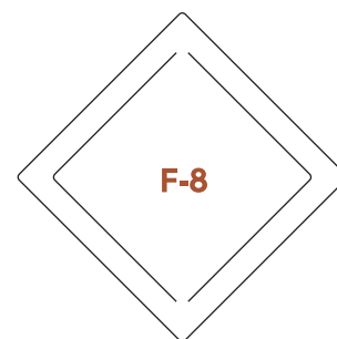
W28×H28mm 0.5R (内刃22mm×22mm)
